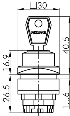
→ Maßskizze
