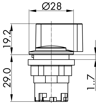
→ Massskizze
