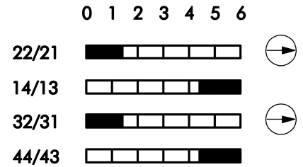
→ Schaltwegediagramm
