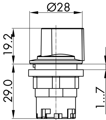
→ Massskizze
