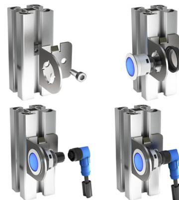
Fig. 4 : Connecteur M12 connect
