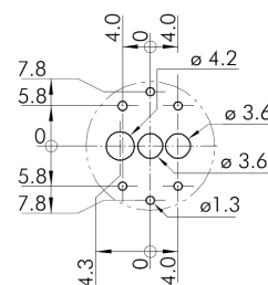
Fig. 2: schéma de montage (FRVKD)
