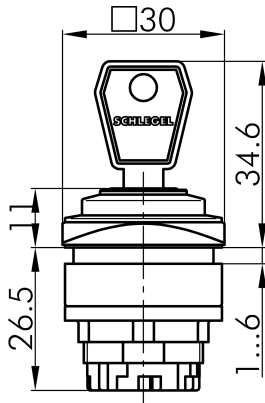
→ Maßskizze
