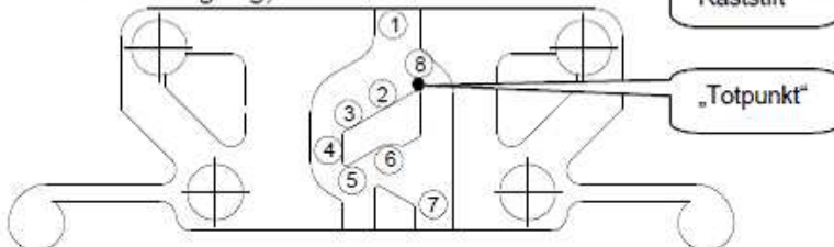
Erneute Betätigung, bevor Raststift in Pos. 1
