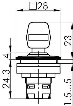
→ Massskizze
