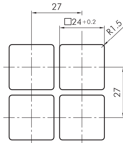
Bohrbild
