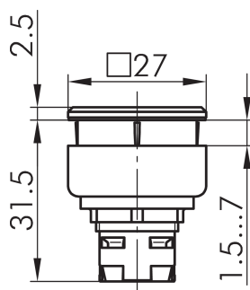
Maßskizze
