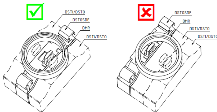
Abbildung 13: DSTOSDE immer in der Mitte montieren
