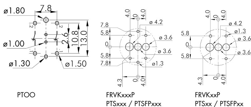
Abbildung 5: Bohrbilder (x ... L, O, I)
