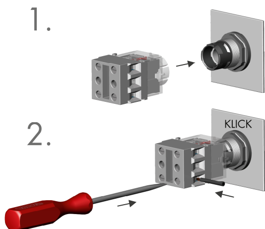
Abbildung 6: Anschluss BTK...
