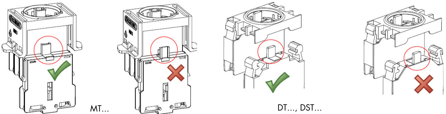
Abbildung 1: Korrekte Montage der modularen Kontaktgeber MT..., DT..., DST...
