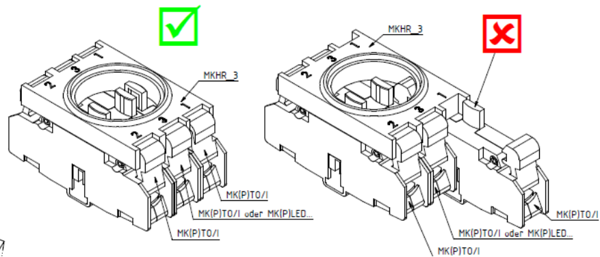
Abbildung 15: Der Stößel darf nicht mit dem Modulhalter MKHR_3 betätigt werden
