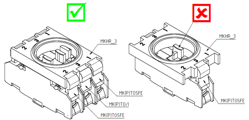
Abbildung 14: MK(P)TOSFE kann auf Position 1 und / oder 2 montiert werden.
