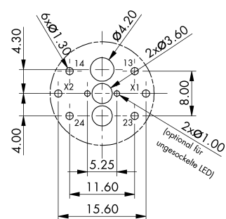
Sicht auf Bestückungsseite der Leiterplatte
