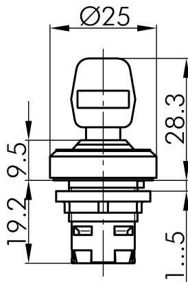
→ Massskizze
