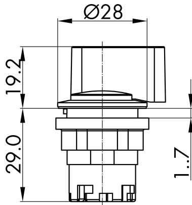
→ Maßskizze
