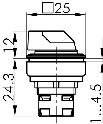
→ Massskizze
