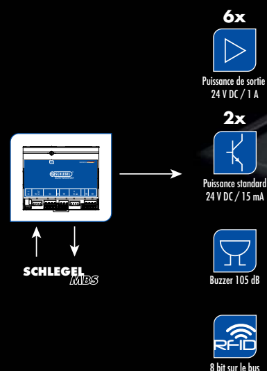
Module d'extension avec commande
