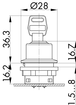
→ Massskizze
