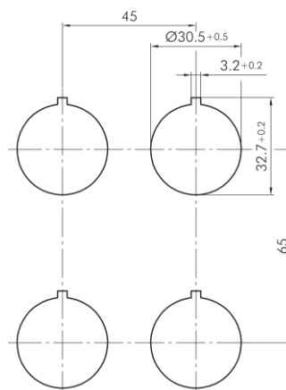
Bohrbild
