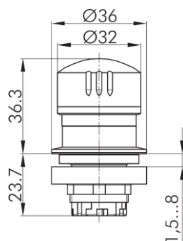
Maßskizze
