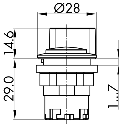
→ Massskizze
