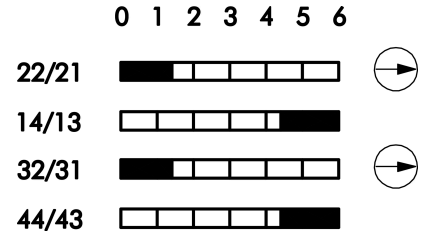
→ Schaltwegediagramm
