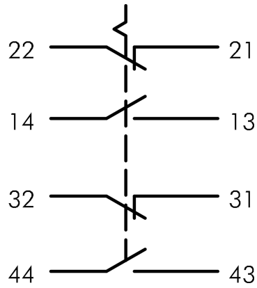
→ Schaltbild
