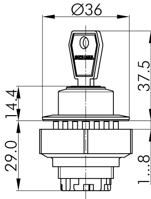
→ Massskizze
