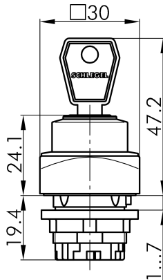
→ Maßskizze
