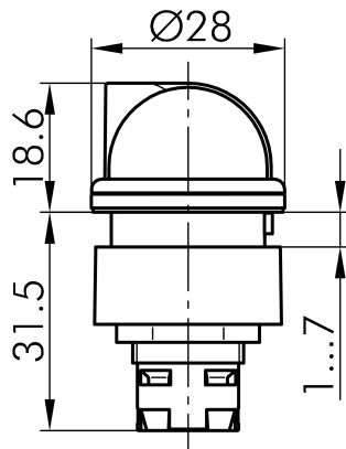
→ Massskizze
