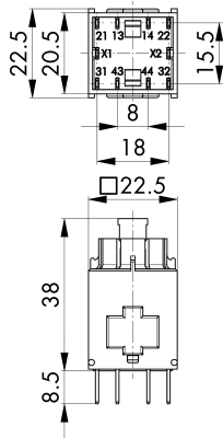
→ Maßskizze
