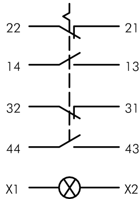
→ Schaltbild
