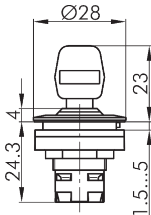
Maßskizze
