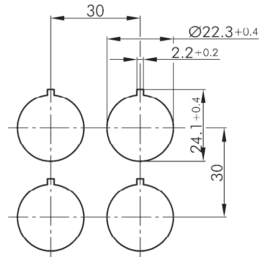
Bohrbild
