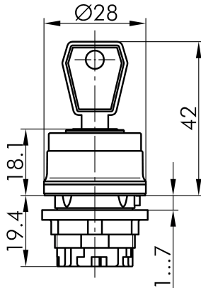
→ Maßskizze
