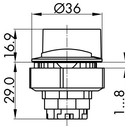
→ Maßskizze
