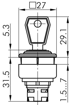
→ Massskizze
