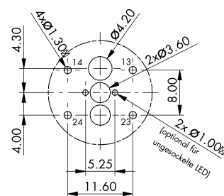
Sicht auf Bestückungsseite der Leiterplatte
