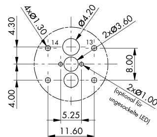
Sicht auf Bestückungsseite der Leiterplatte
