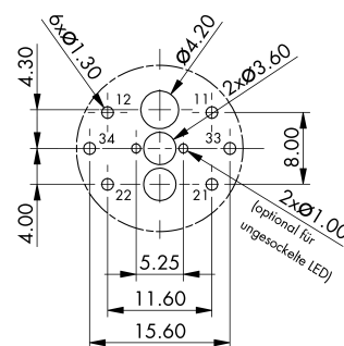
Sicht auf Bestückungsseite der Leiterplatte
