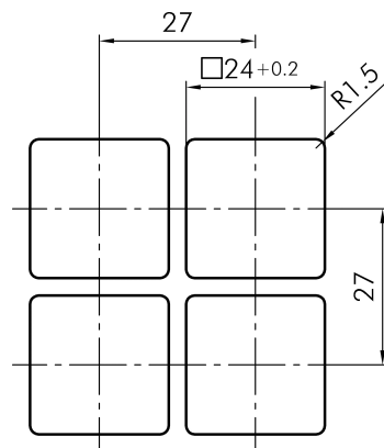
→ Bohrbild
