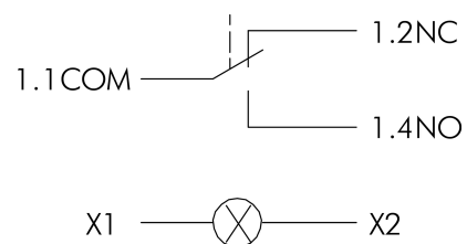
→ Schaltbild
