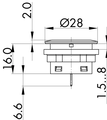
→ Maßskizze
