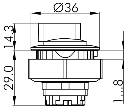
→ Massskizze
