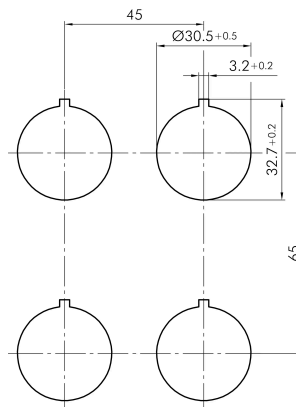
→ Bohrbild
