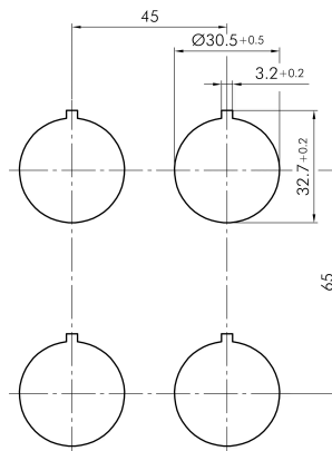
→ Bohrbild
