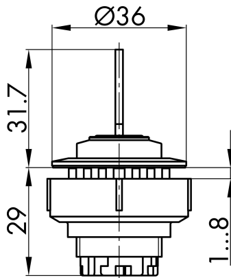
→ Massskizze
