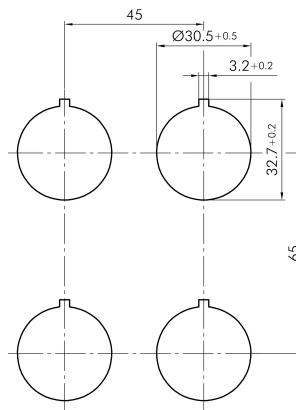
→ Bohrbild
