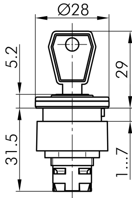
→ Massskizze
