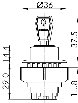
→ Massskizze
