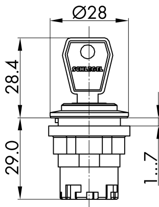
→ Maßskizze
