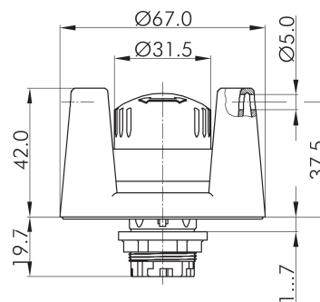
Maßskizze
