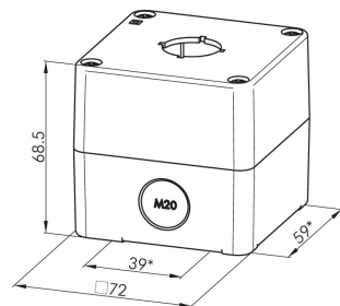
Maßskizze
