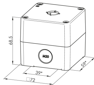
Maßskizze
