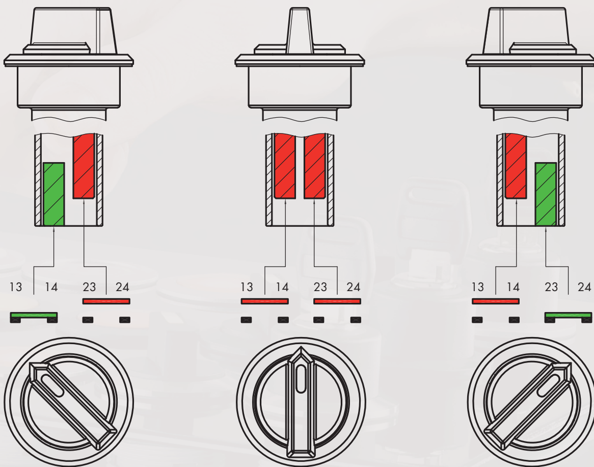
Abbildung zweigeteilter Stößel
