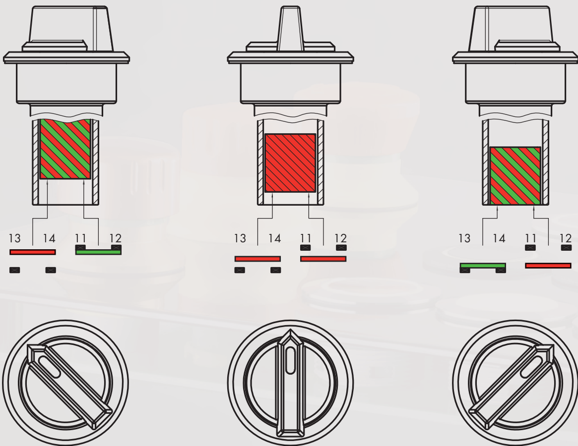
Abbildung einteiliger Stößel
